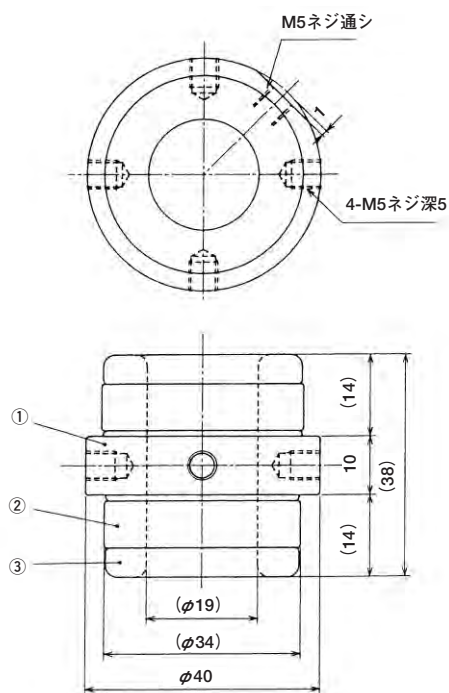
シリコンエアグリッパー製品図 (G020GSFX100)
